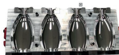
Soufflage PET
